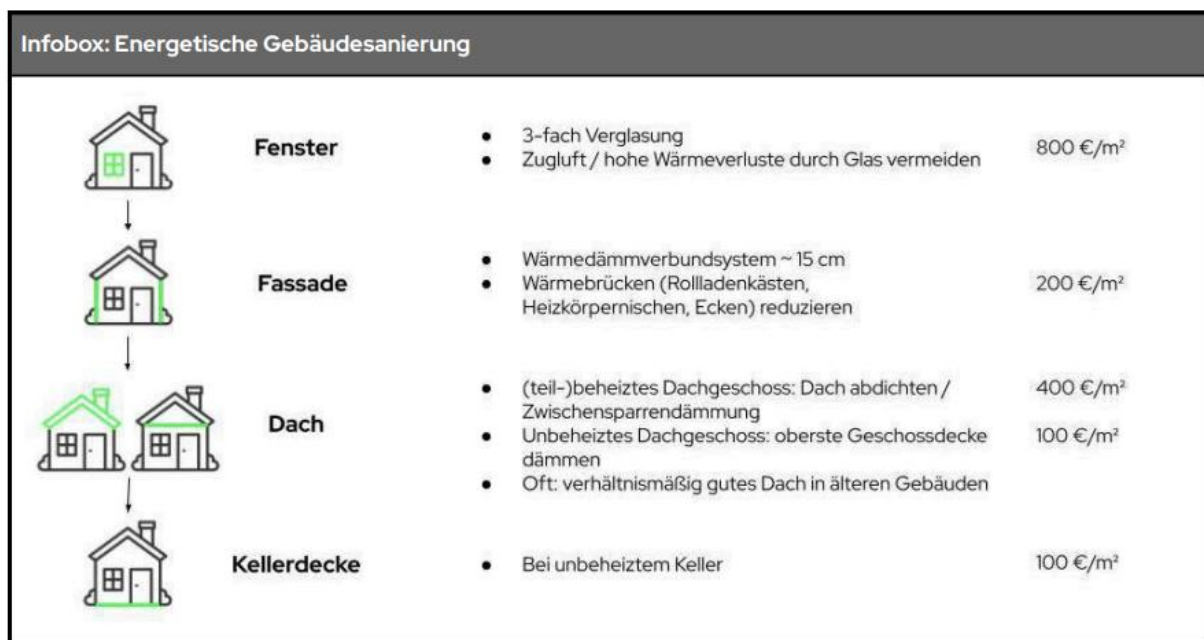
Abbildung 19: Energetische Gebäudesanierung
