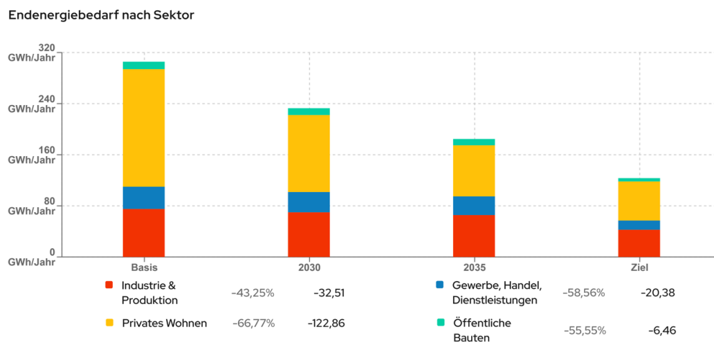
Abbildung 42: Endenergiebilanz Status Quo und für das Zielszenario der Jahre 2030,2035 und 2040 nach Sektoren
