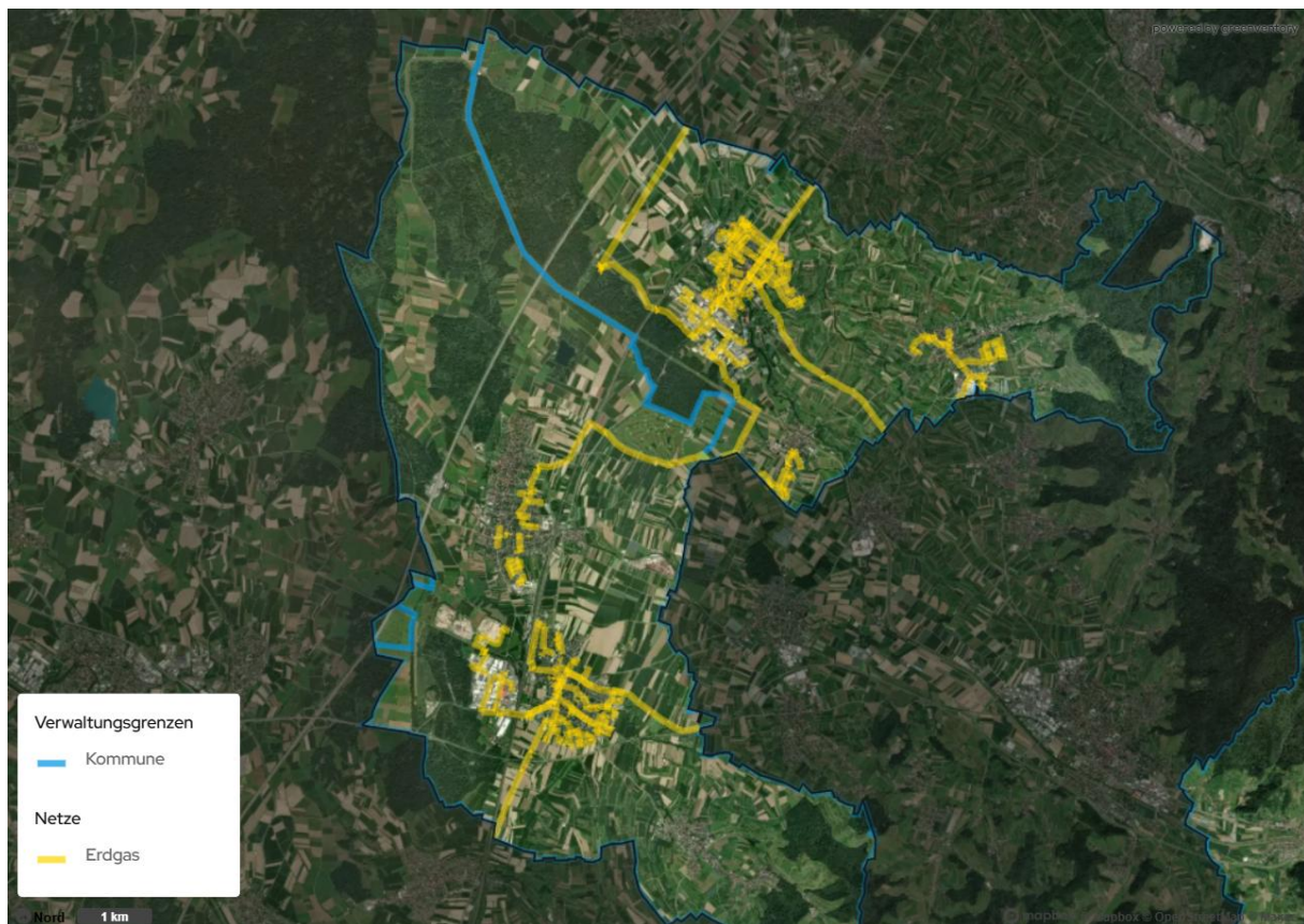
Abbildung 12: Gasnetze Appenweier und Renchen
