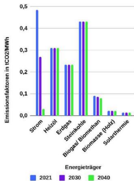
Abbildung 47: Emissionsfaktoren in tCO 2 /MWh
