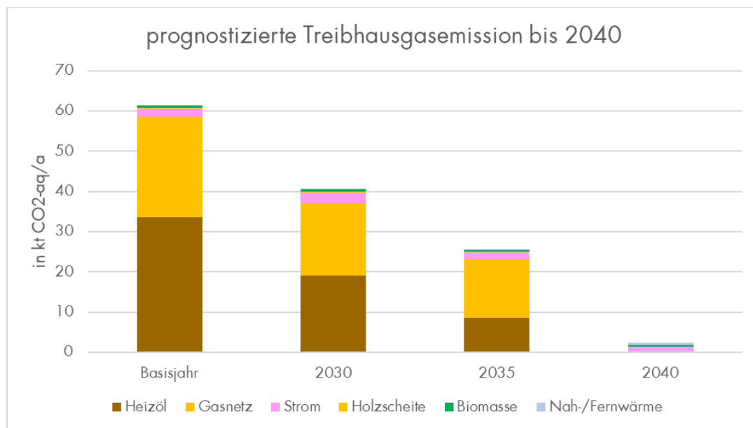
Abbildung 46: Treibhausgasbilanz Status Quo u. für die Zielszenarien der Jahre 2030,2035 und 2040
