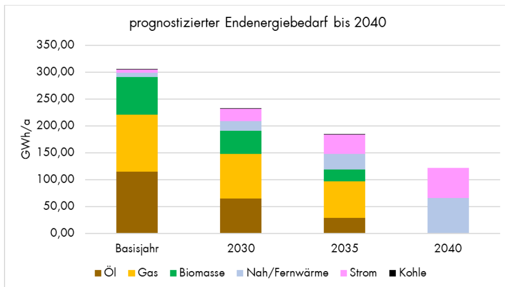
Abbildung 41: Endenergiebilanz Status Quo und für das Zielszenario der Jahre 2030,2035 und 2040 nach Energieträger
