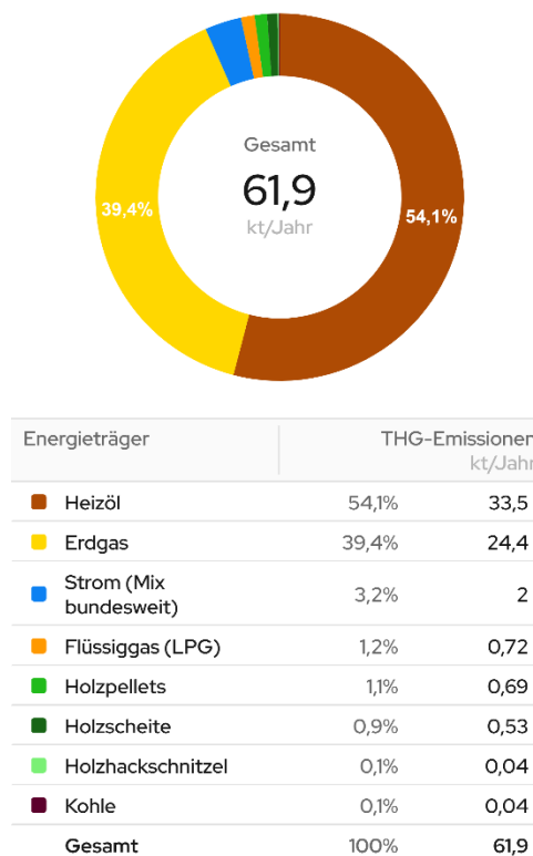
Abbildung 14: Treibhausgas Verteilung
